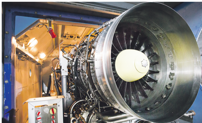
Уфимский двигатель АЛ-31 СТ производства ПАО «ОДК-УМПО» – в авангарде импортозамещающей продукции региона для газовой отрасли
