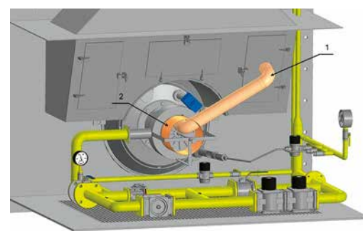
Система рециркуляции дымовых газов (РДГ) 1 – воздухопровод; 2 – зона смешения
